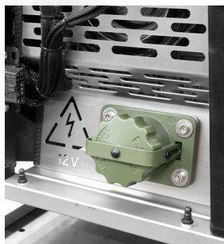
NATO-Fremdstartsteckdose 12 V DC und OBD II Diagnosestecker
